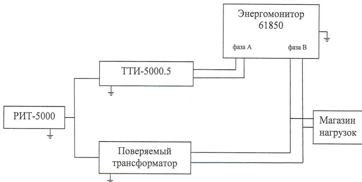
Рисунок 2 – Схема определения погрешностей коэффициента масштабного преобразования, угла фазового сдвига (для трансформаторов классов точности ТРХ; ТРУ; ТРZ) и погрешности по виткам (для трансформаторов классов точности РХ; РХR)
