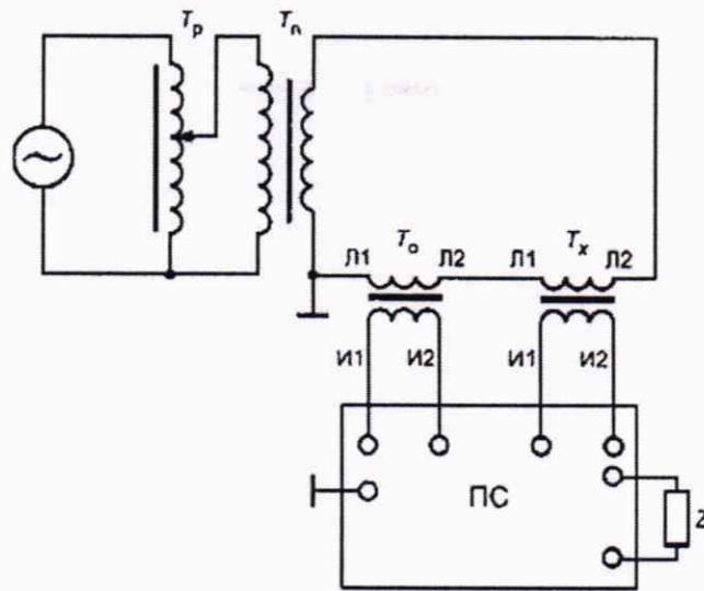
\sim – сеть (генератор); T_p – регулирующее устройство (автотрансформатор); T_n – понижающий силовой трансформатор; T_o – рабочий эталон; T_x – поверяемый трансформатор тока; L_1, L_2 – контактные зажимы первичной обмотки; I_1, I_2 – контактные зажимы вторичной обмотки; Z – нагрузка (схема подключения нагрузки зависит от прибора сравнения и указывается в эксплуатационной документации на прибор сравнения); ПС – прибор сравнения Рисунок 2 – Схема поверки с использованием рабочего эталона и прибора сравнения (компаратора вторичных токов)
