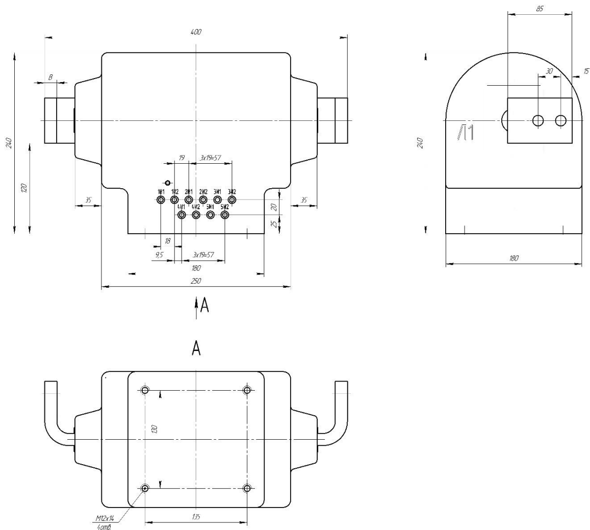
Рис.1 Общий вид трансформатора ТЛП-5 на токи 1000-1500А.
