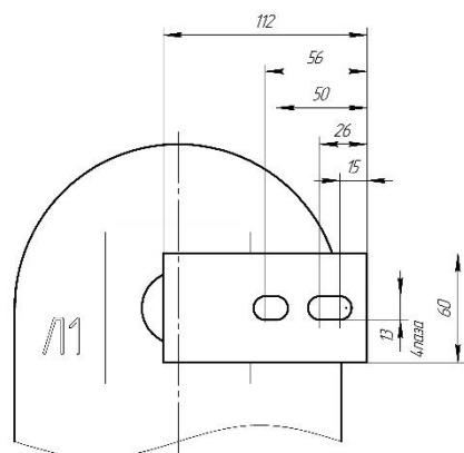
Рис.2 Общий вид трансформатора ТЛП-5 на ток 2000А. Остальное см. на рис.1
